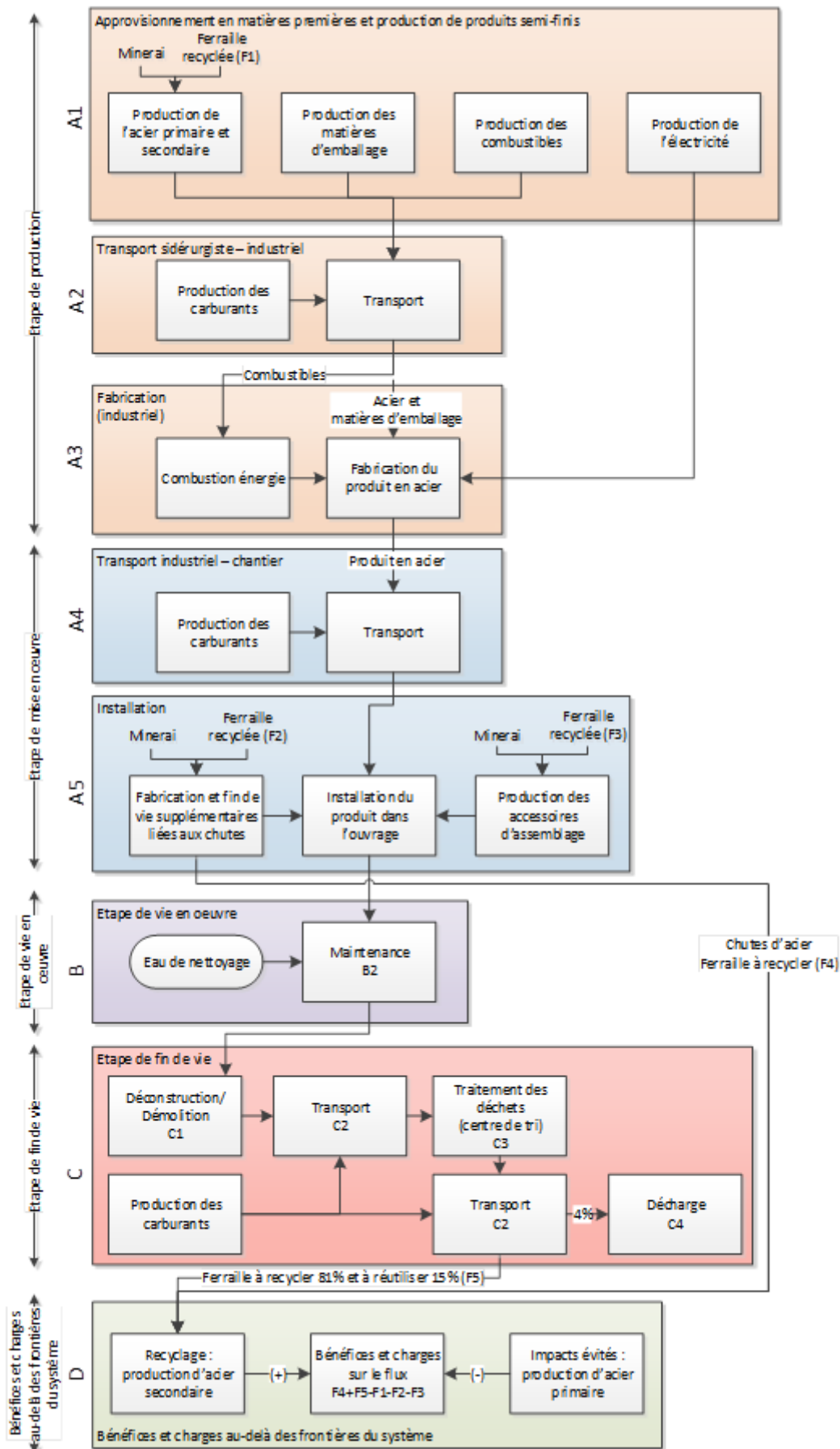
- Cycle de vie du produit en acier
